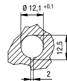
Einbauöffnung mounting hole trou de montage
